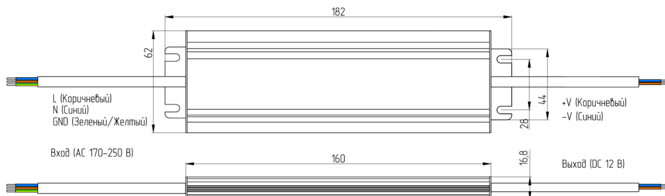
Рисунок 2 – Габаритный чертеж.
