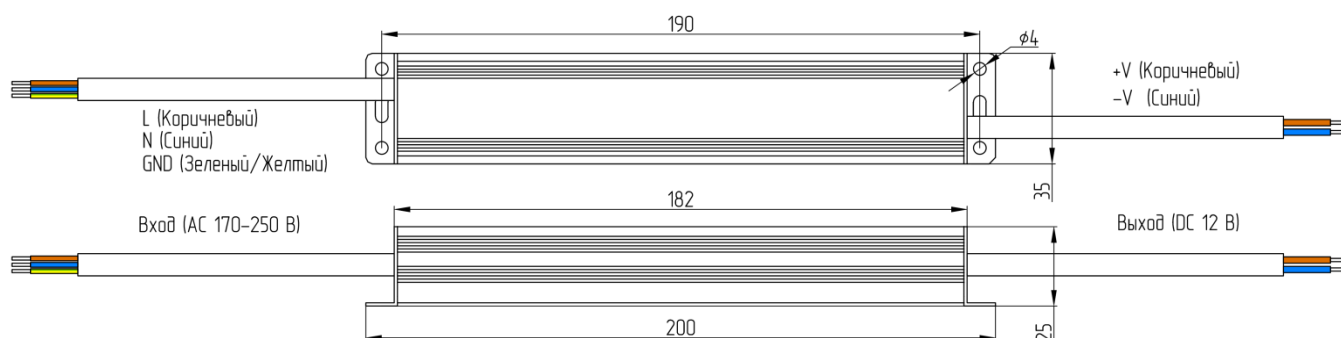
Рисунок 2 – Габаритный чертеж.
