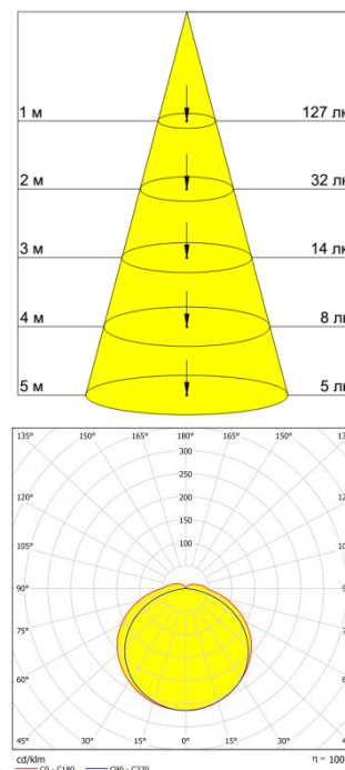
Рисунок 3 – Светораспределение светильника Geniled Лайнер-Т 8W 5000К.
