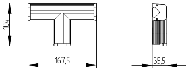
Рисунок 2 – Габаритные размеры светильника Geniled Лайнер-Т 8W 5000К.
